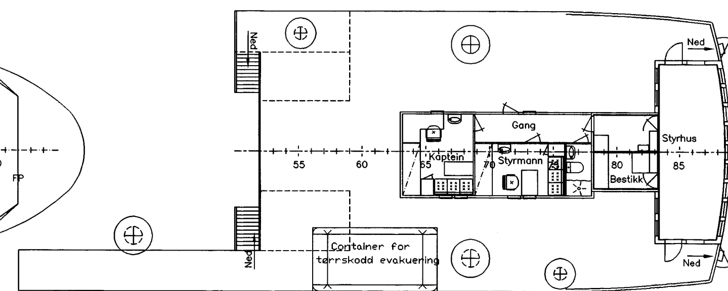
Brodekk
