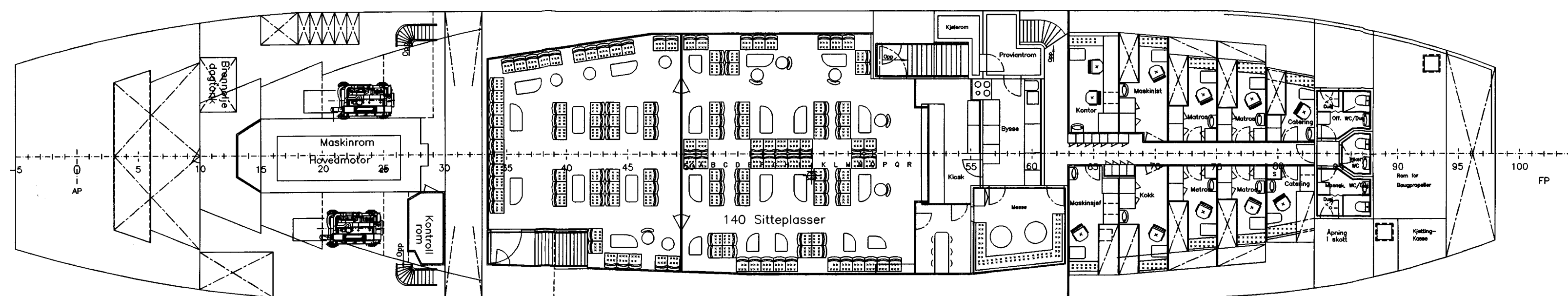
Snitt under hoveddekk
