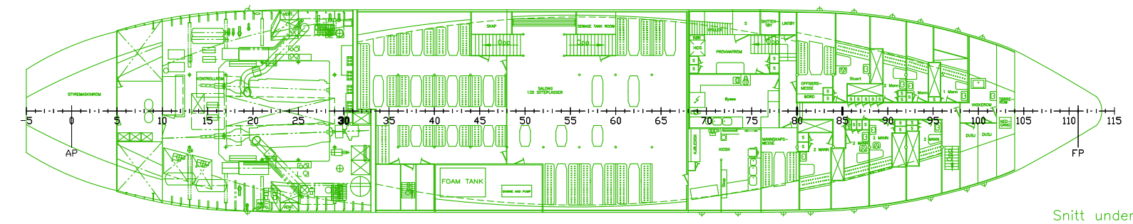
Snitt under hoveddekk
