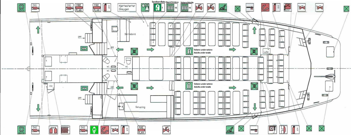
PLAN HOVEDDEK
