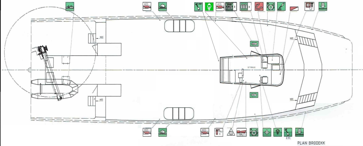
PLAN BRØDEDEK
