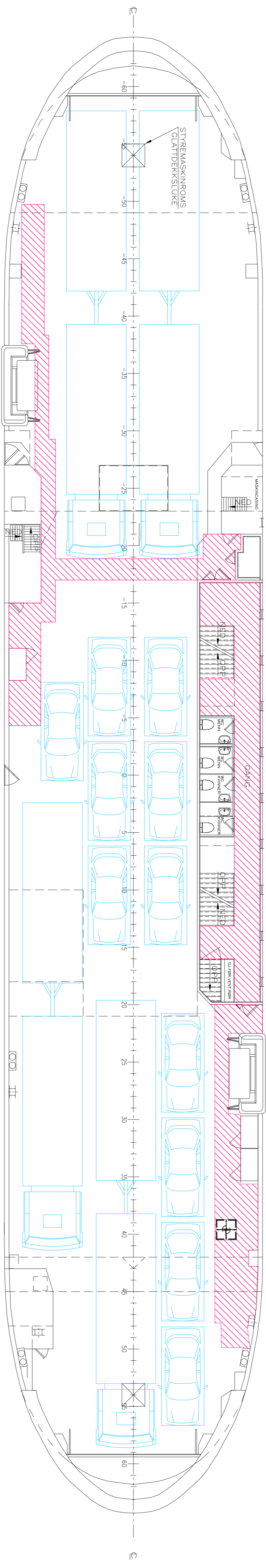
HOVEDDEKK - KOMBINERTLAST 11 PER, 4 VTE
